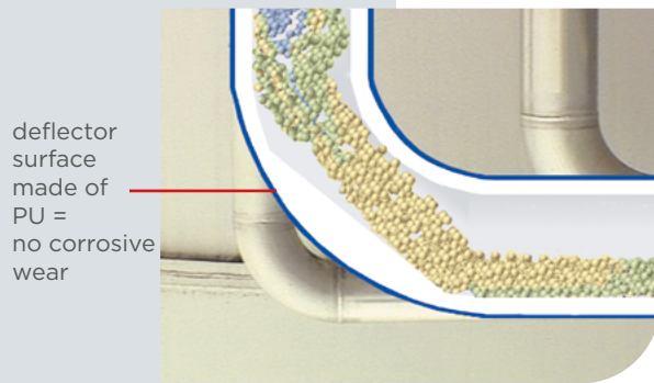
Master-PROTECT Pipe-Bend
