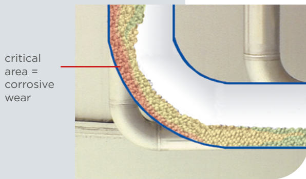
Standard Pipe-Bend
